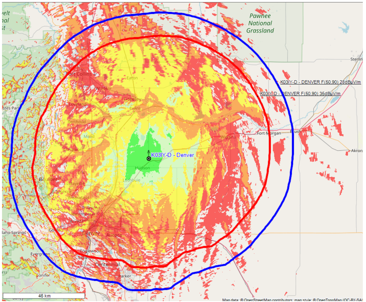
Рисунок 49. Контуры FCC
