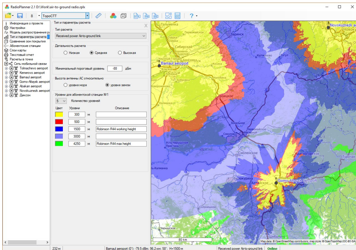
Рисунок 54. Пример расчета для зоны покрытия для малой авиации
