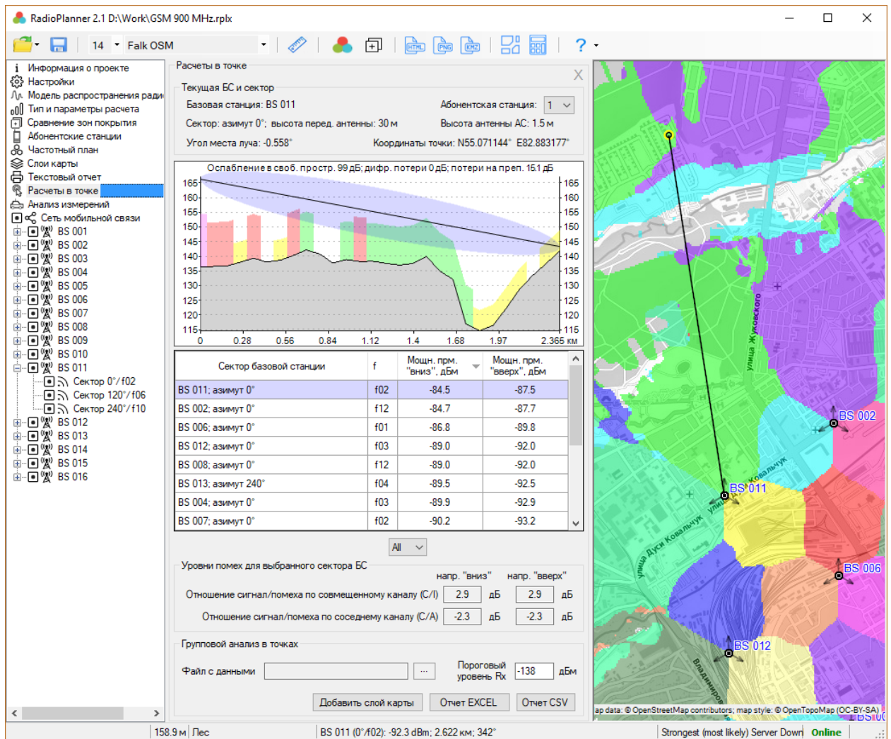
Рисунок 33. Расчеты в точке
