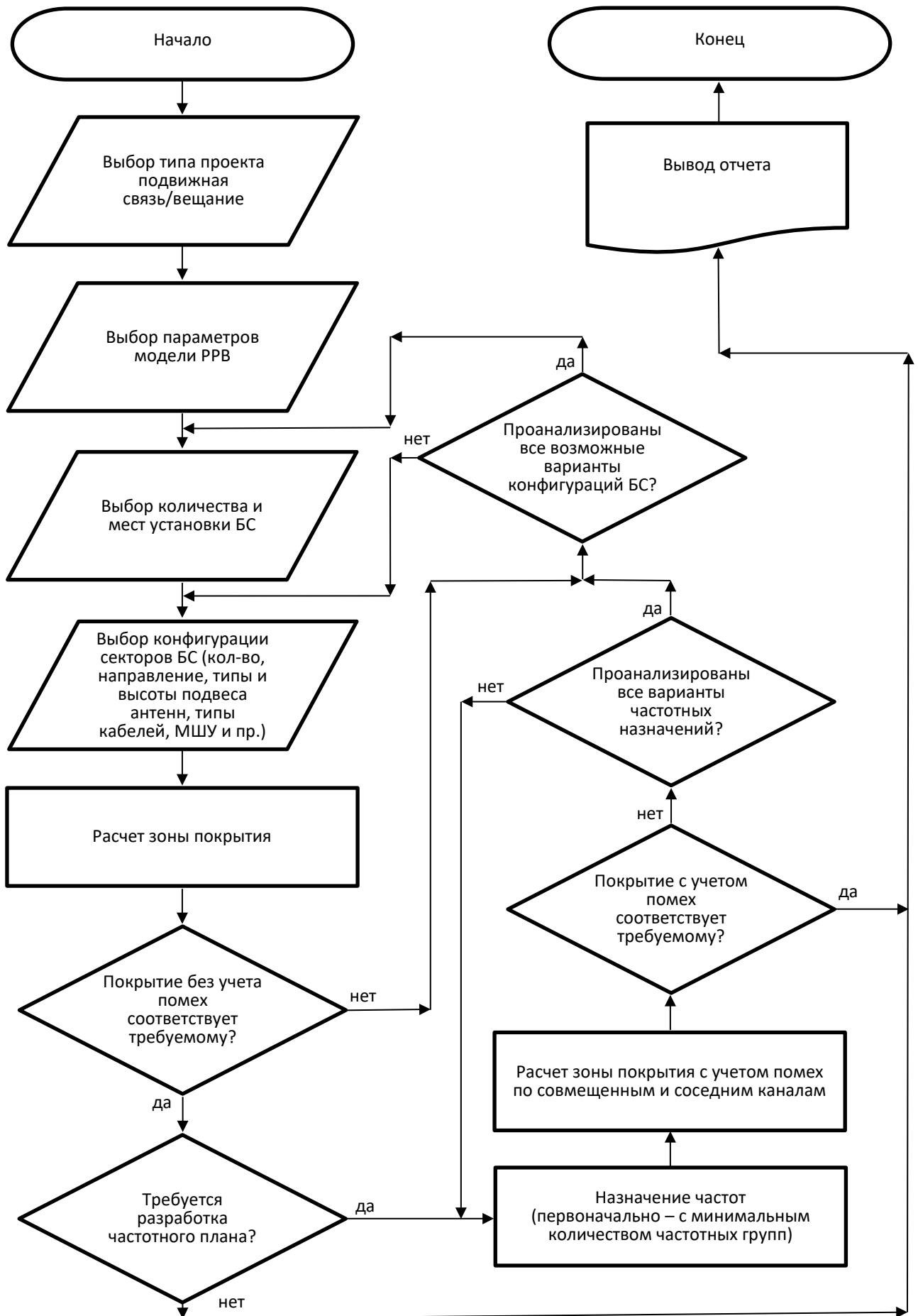
Рисунок 15. Общая блок-схема алгоритма работы с программой RadioPlanner
