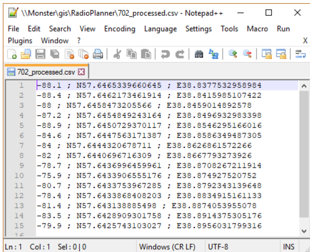
Рисунок 5. Пример текстового файла в формате CSV с результатами измерений
