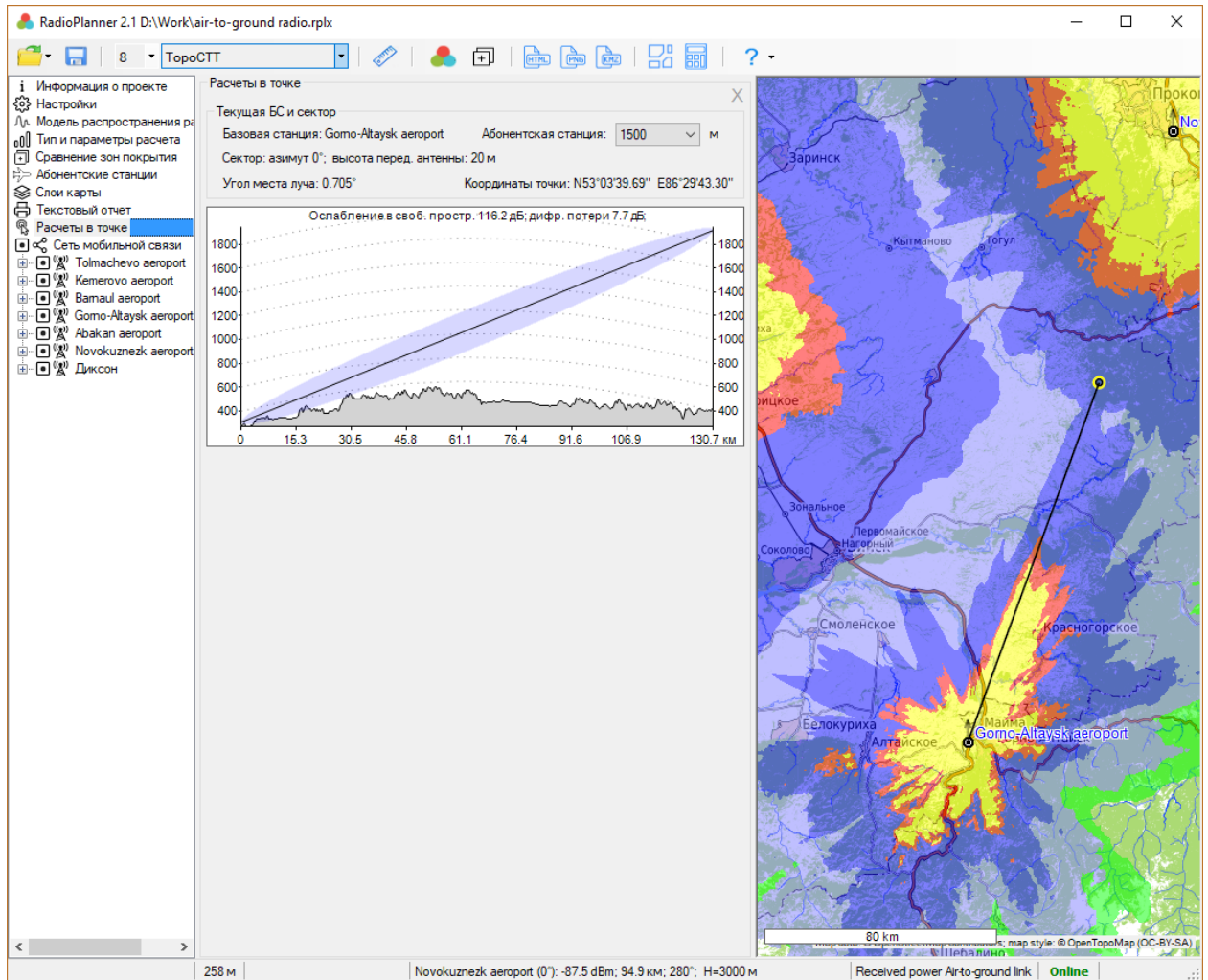
Рисунок 58. Расчеты в точке для авиационной радиосвязи
