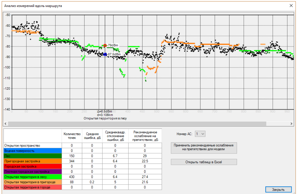
Рисунок 40. Анализ измерений вдоль маршрута
