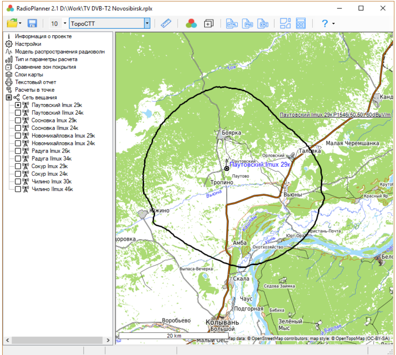
Рисунок 50. Контур по МСЭ-R P.1546-6
