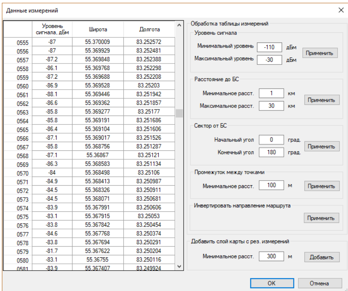
Рисунок 39. Предварительная обработка результатов измерений в секторе БС
